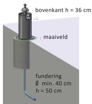
8.30.6.1 Waterdispenser met fundering (incl. bodemkoker)
