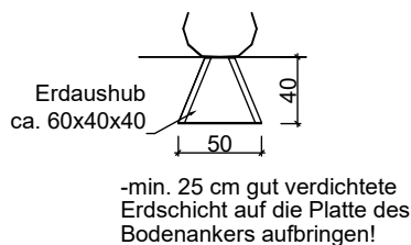
Bodenanker 11.1.5.2
