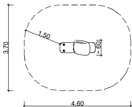
Draufsicht mit Mindestraum M 1:100 m,cm
