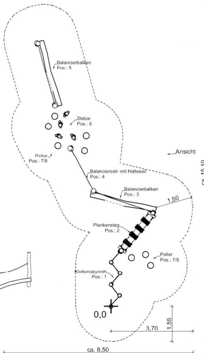
Bovenaanzicht
